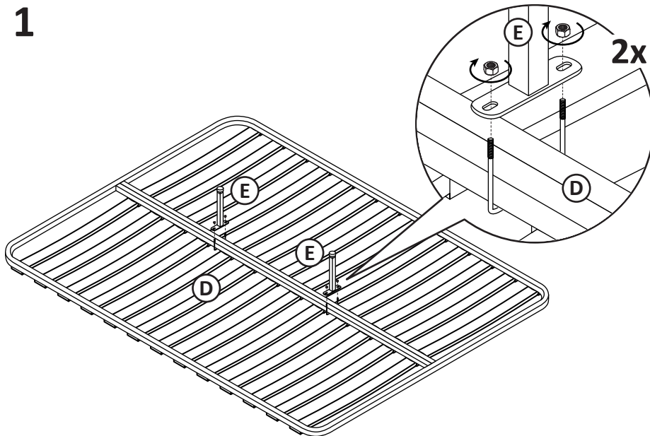
E - Leg x 2
