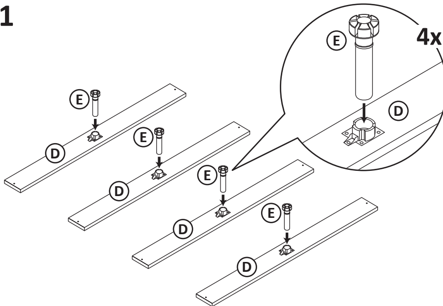
E - Leg x 4
